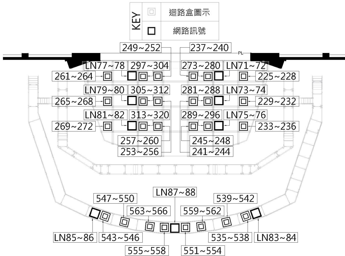
圖例 2.3.5 張力索棚架與貓道迴路配置
