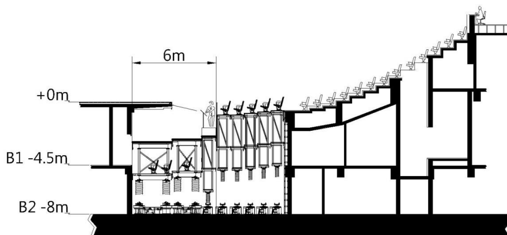
圖例 1.2.1.2-樂池升降平台剖面圖
