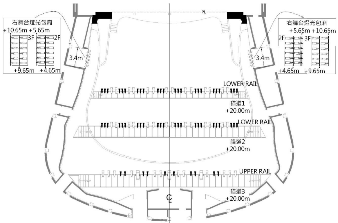
圖例 2.1 外區燈具配置圖
