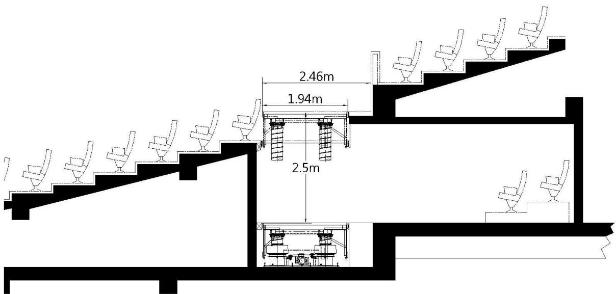
圖例 1.2.2.2-觀眾席控制區升降平台位置圖
