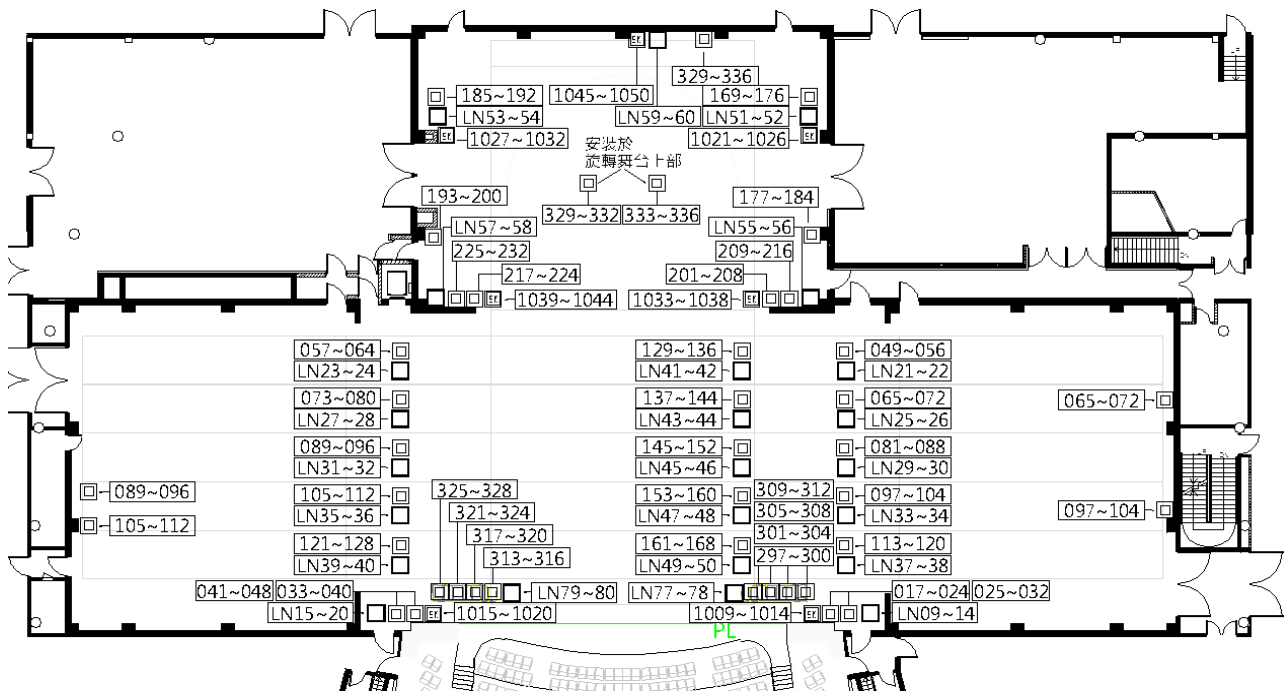
圖例 2.3.1.1-一樓燈光迴路配置圖
