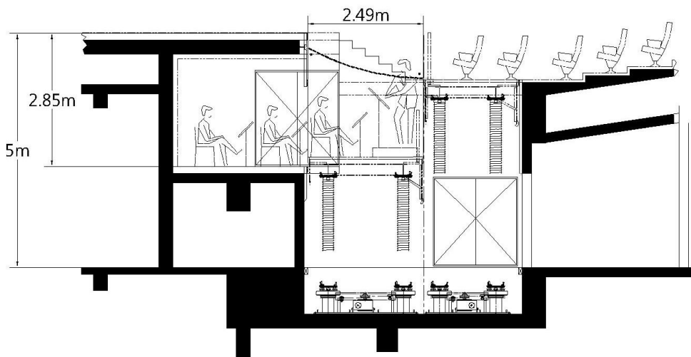
圖例 1.2.1.2-樂池立面圖
