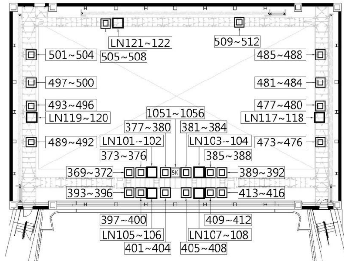
圖例 2.3.1.3-三樓廊道及燈光橋燈光迴路配置圖
