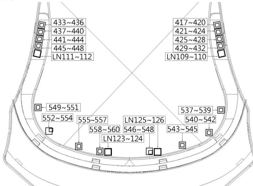
圖例 2.3.2.3- 三樓樓座前緣及燈光包廂燈光迴路配置圖
