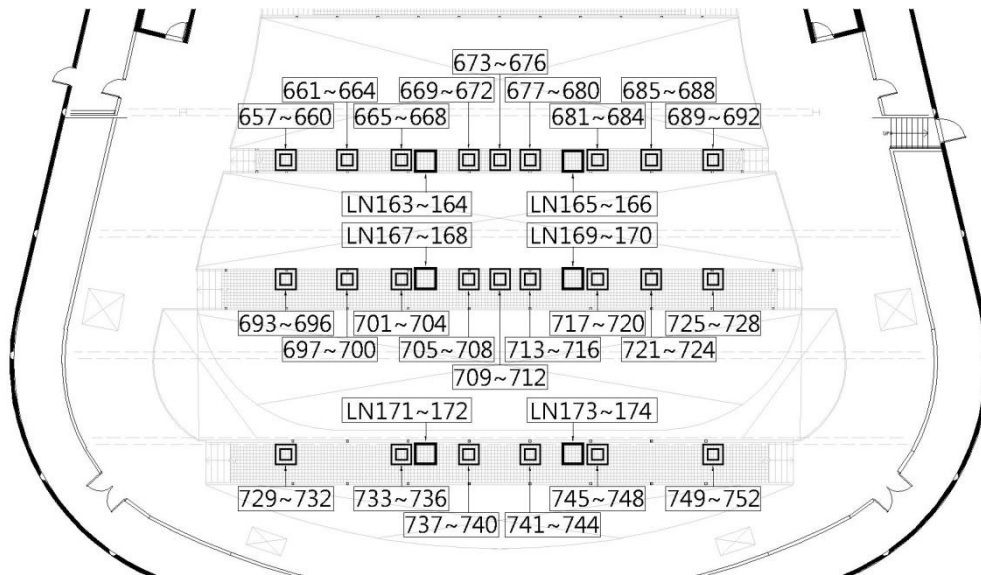
圖例 2.3.2.3- 三樓樓座前緣及燈光包廂燈光迴路配置圖
