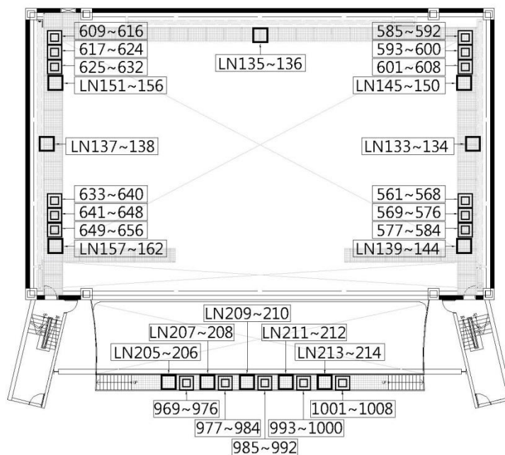
圖例2.3.1.4-四樓廊道燈光迴路配置圖
