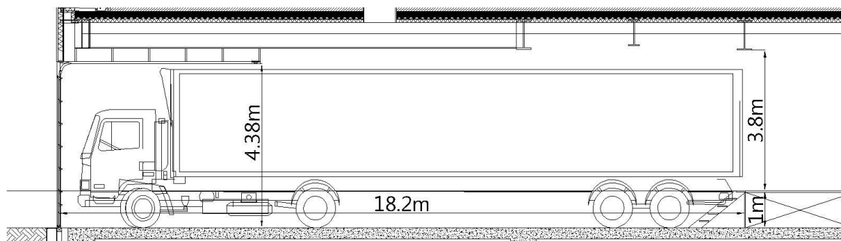
圖例 4.2 西碼頭卸貨口剖面圖
