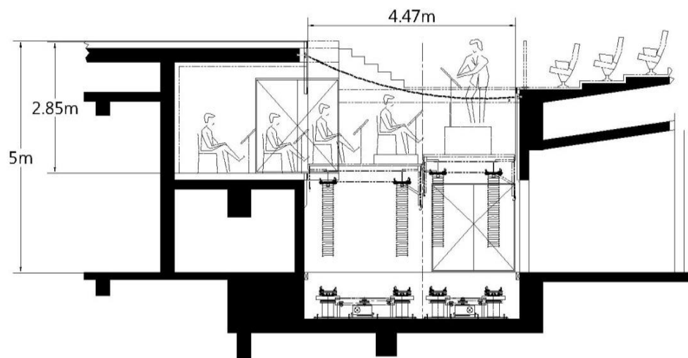
圖例 1.2.1.3-樂池立面圖
