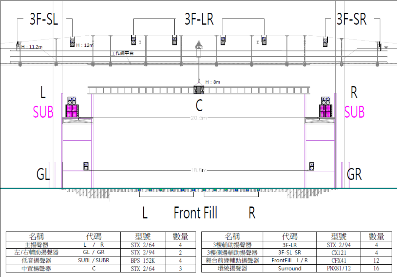
圖例 4-1.1 揚聲器配置立面圖
