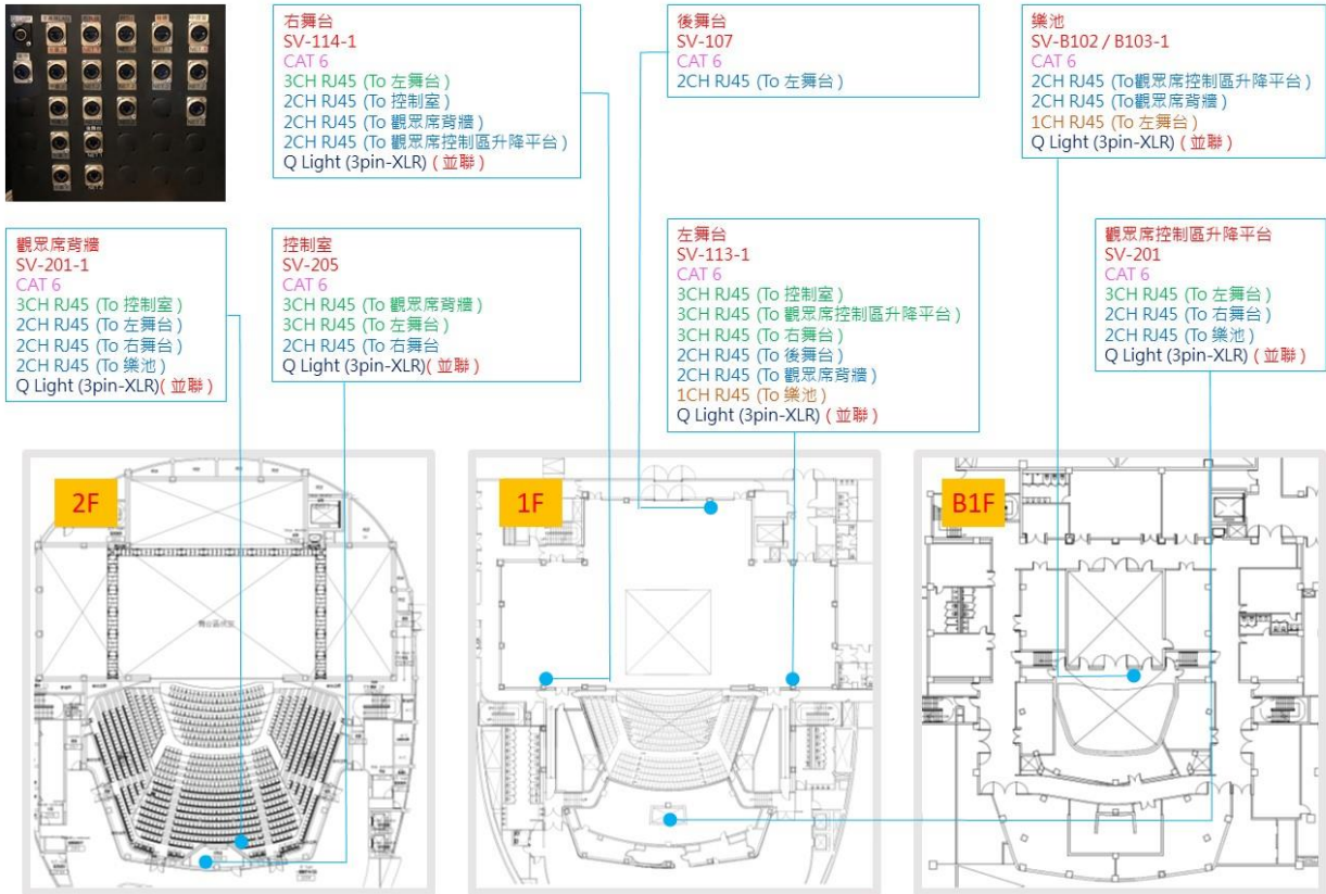
圖例 4-1.8 RJ45 信號通道圖示
