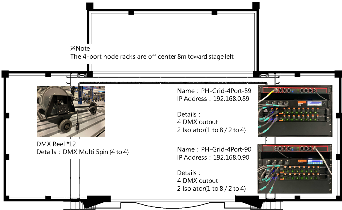
圖例 3.3.1- 頂棚區 Node 位置圖
