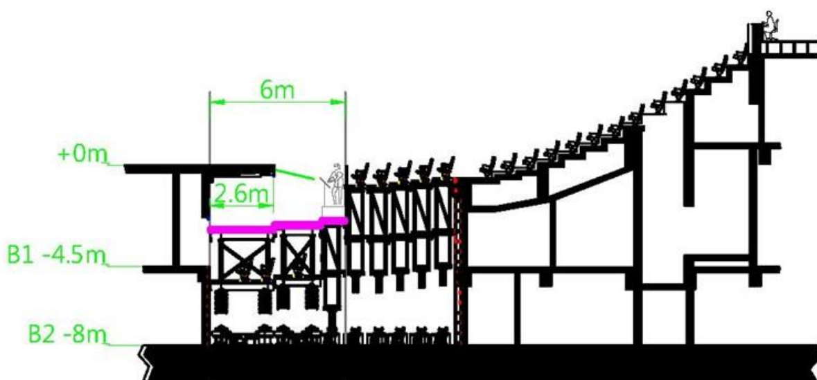
圖例 122.1.2-樂池升降平台剖面圖
