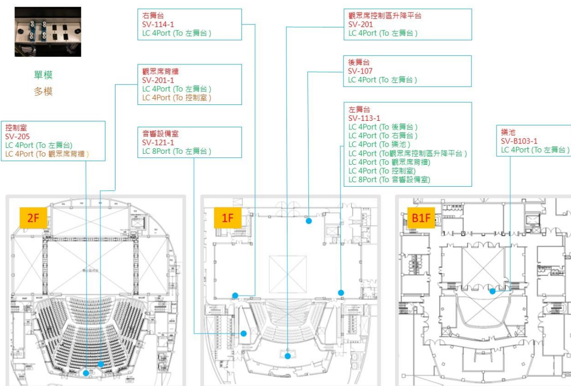
圖例 4-1.6 光纖通道圖示
