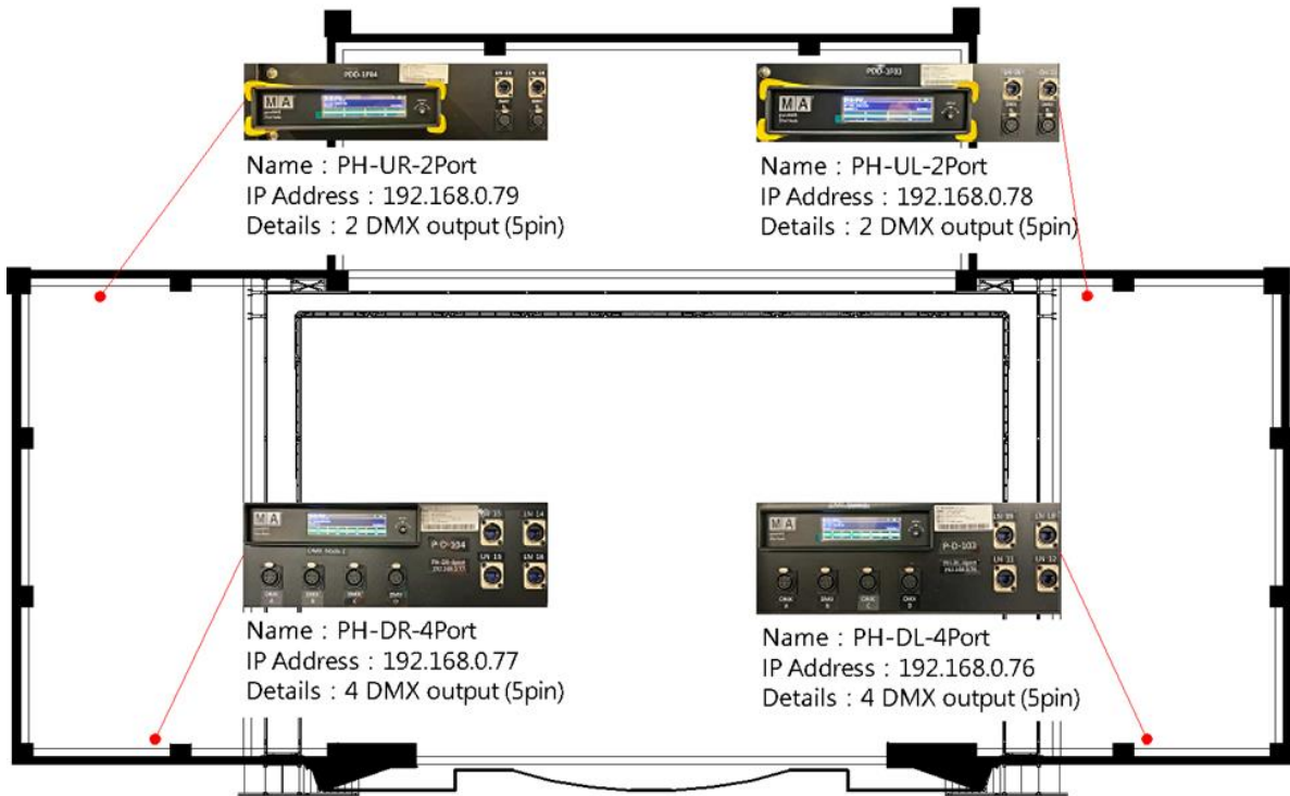
圖例 3.3.2- 舞台區 Node 位置圖
