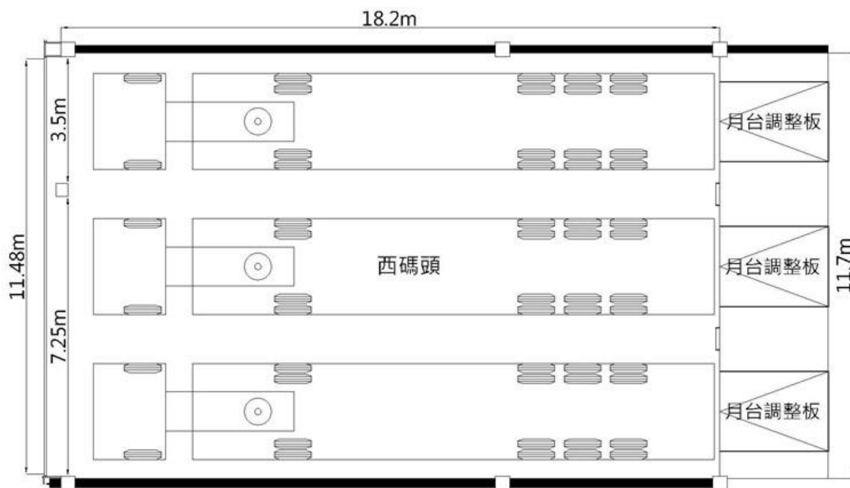
圖例 5.1 西碼頭卸貨口平面圖
