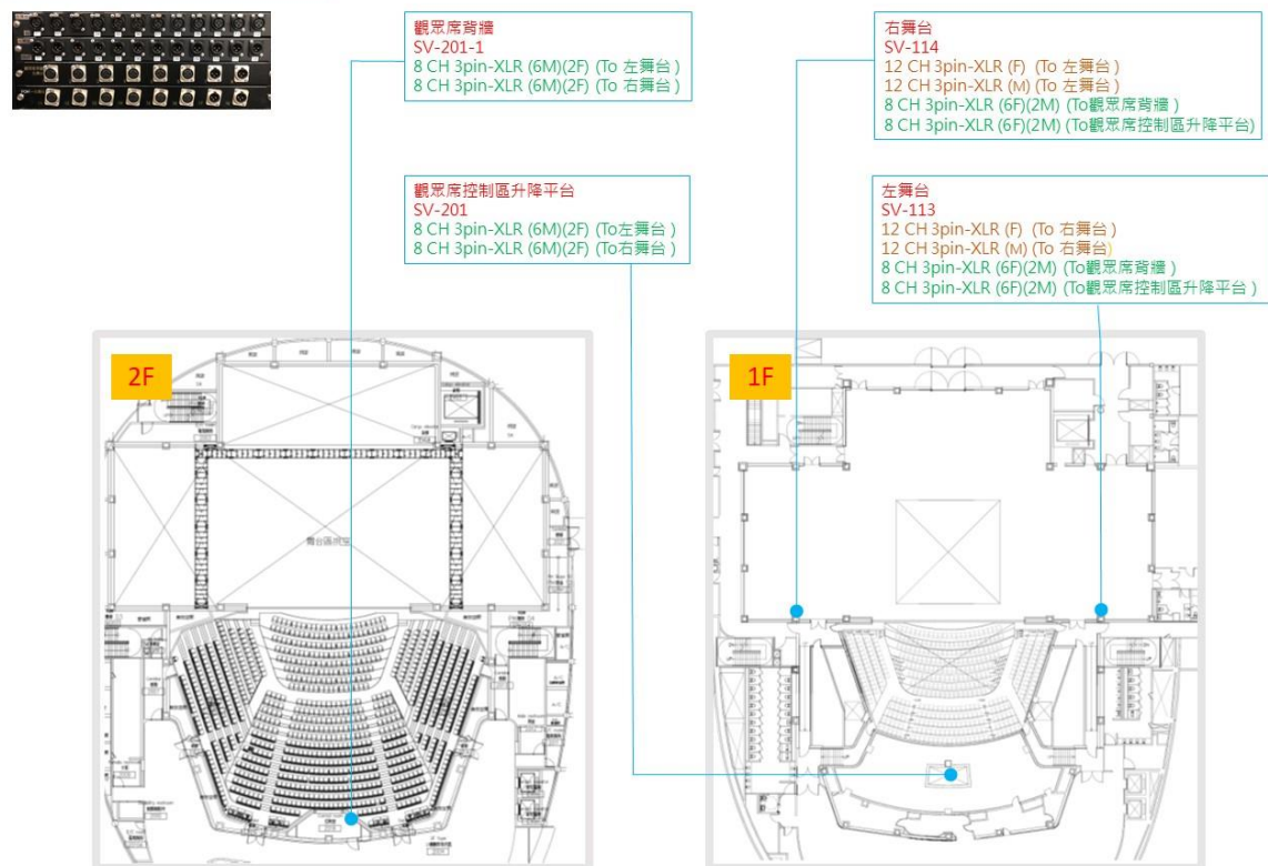
圖例 4-1.7 信號通道圖示
