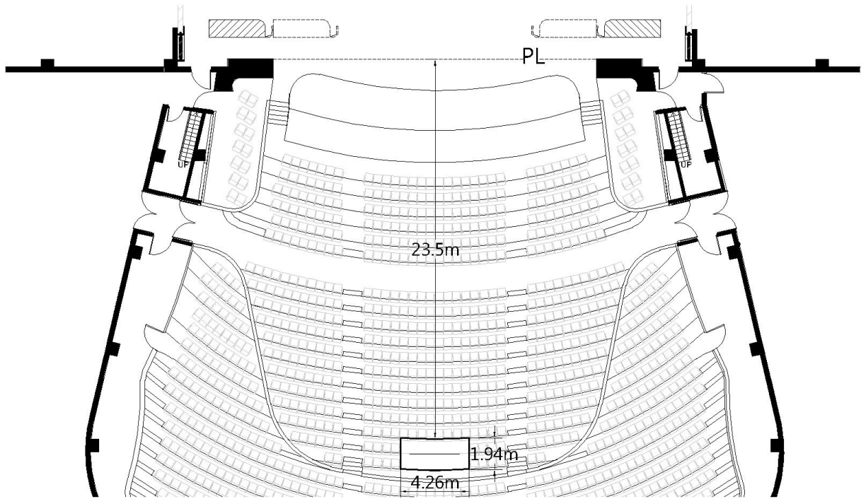
圖例 1.2.2.1-觀眾席控制區升降平台位置圖
