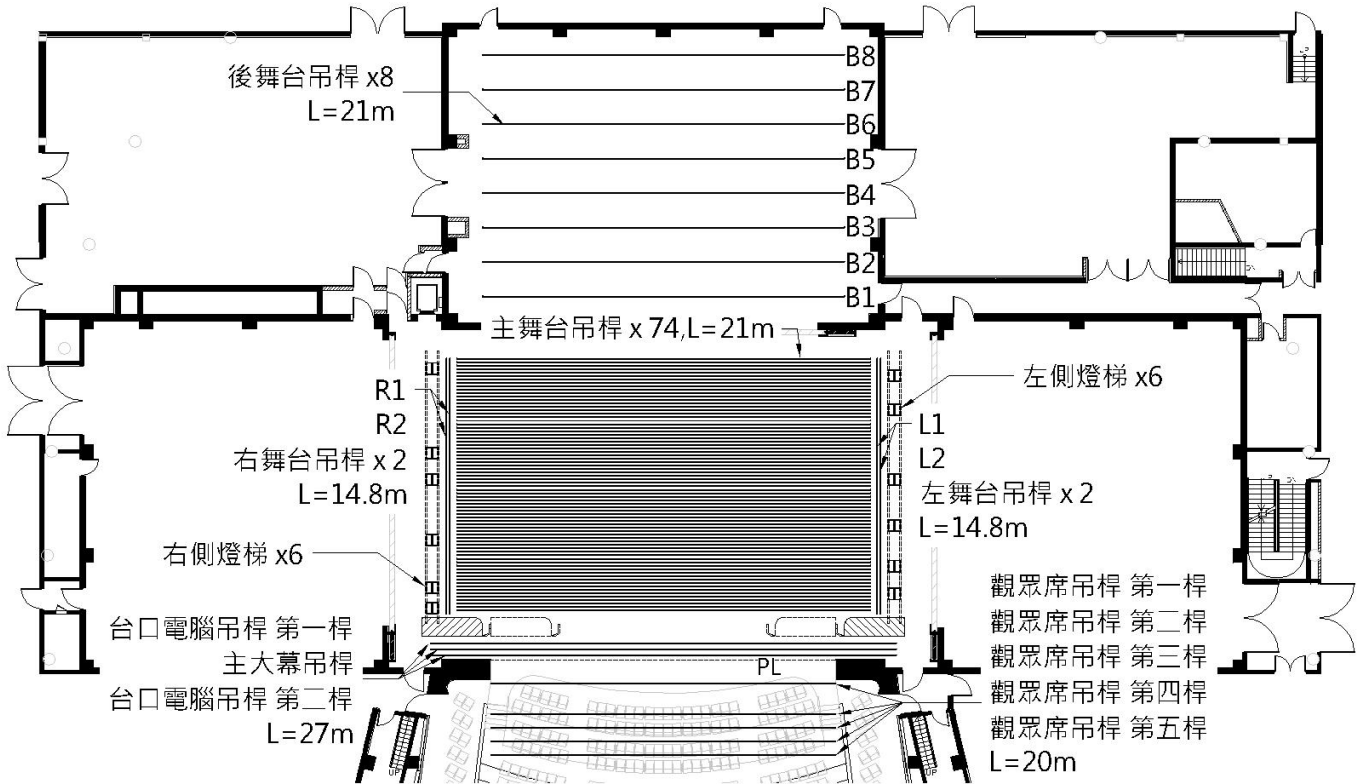
圖例 1.3.1-吊桿平面圖
