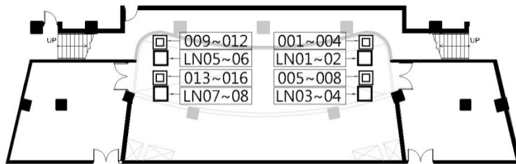
圖例 2.3.2.1-樂池升降平台燈光迴路配置圖
