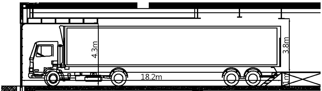
圖例 4.2 西碼頭卸貨口剖面圖
