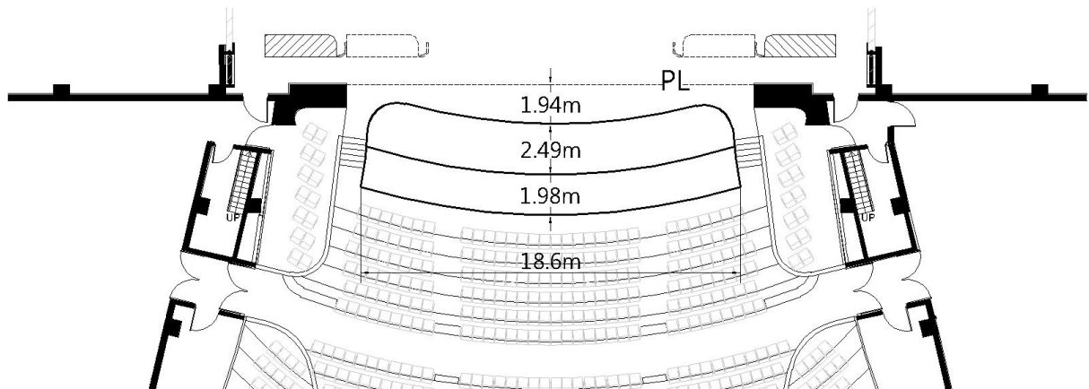
圖例 1.2.1.1-樂池升降平台位置圖
