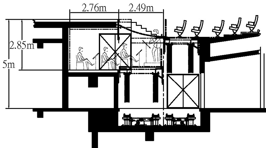
圖例 1.2.1.2-樂池立面圖
