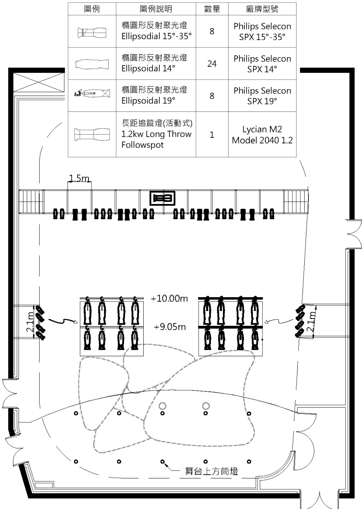
圖例 2.1 燈具配置圖
