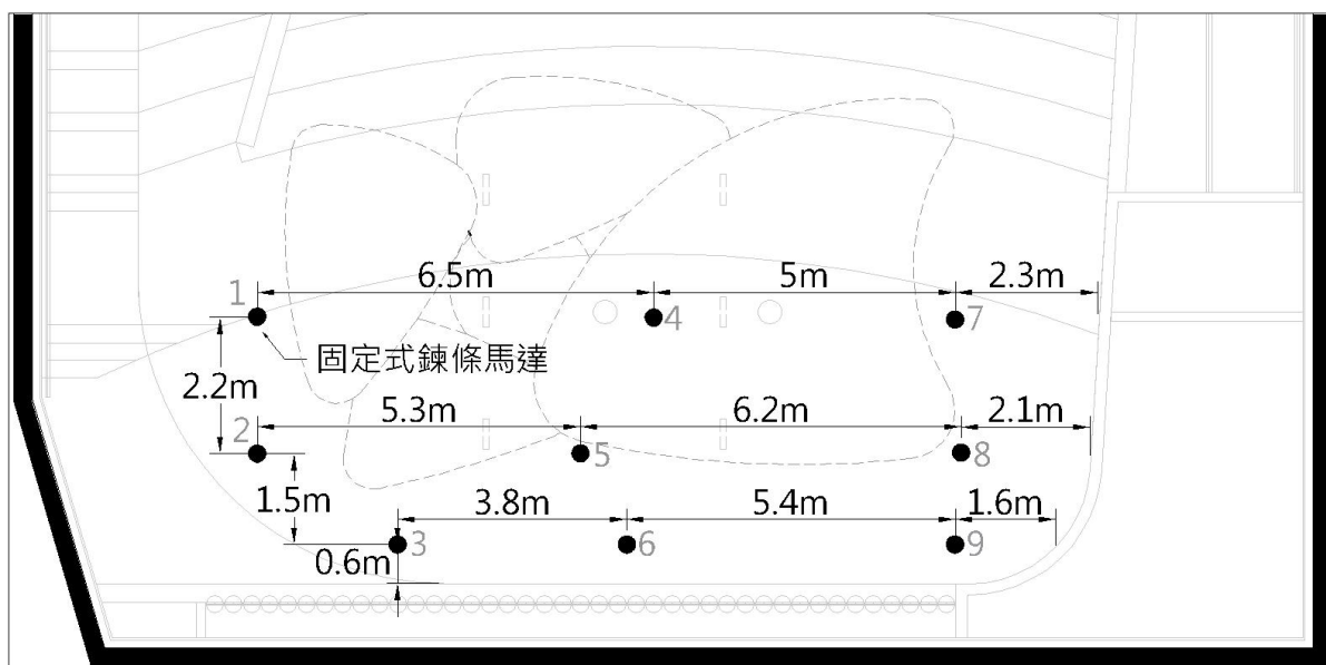
圖例 1.4 鍊條吊車位置圖
