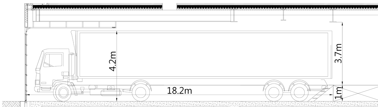
圖例 4.2 西碼頭卸貨口剖面圖
