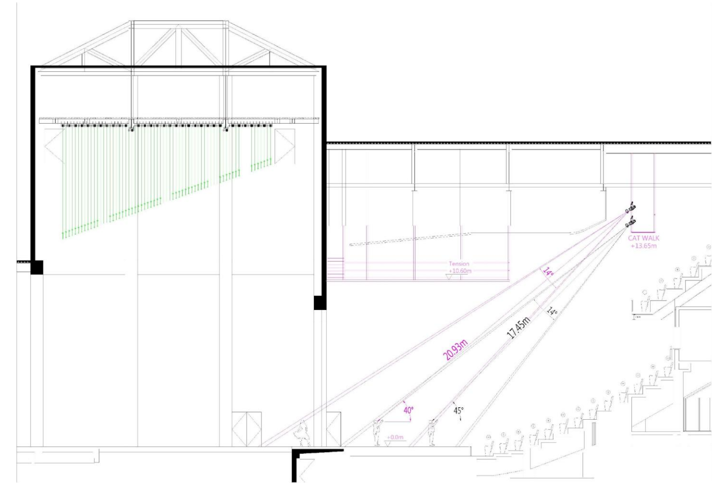
圖例 3.2.2- 外區燈光剖面圖
