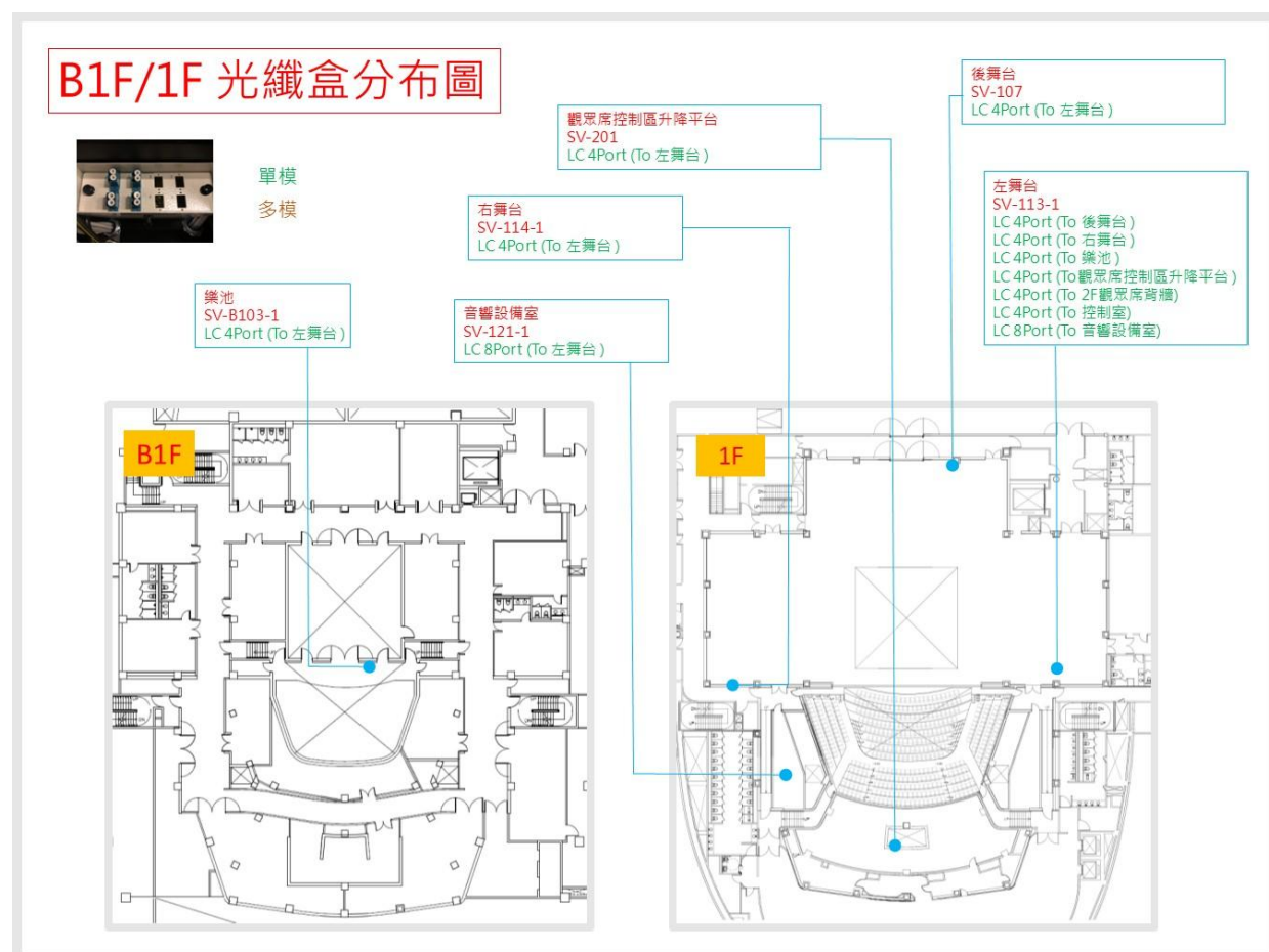
圖例 4-1.6 B1F/1F 光纖通道圖示
