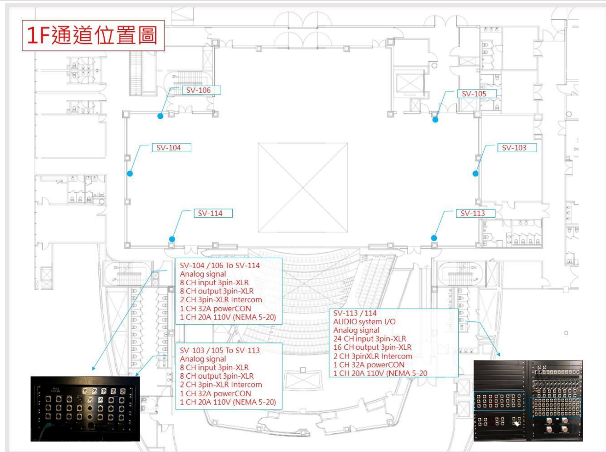
圖例 4-1.3 音響 1F 通道圖示
