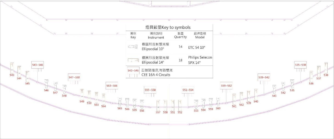
圖例 3.2.1- 外區燈具配置圖
