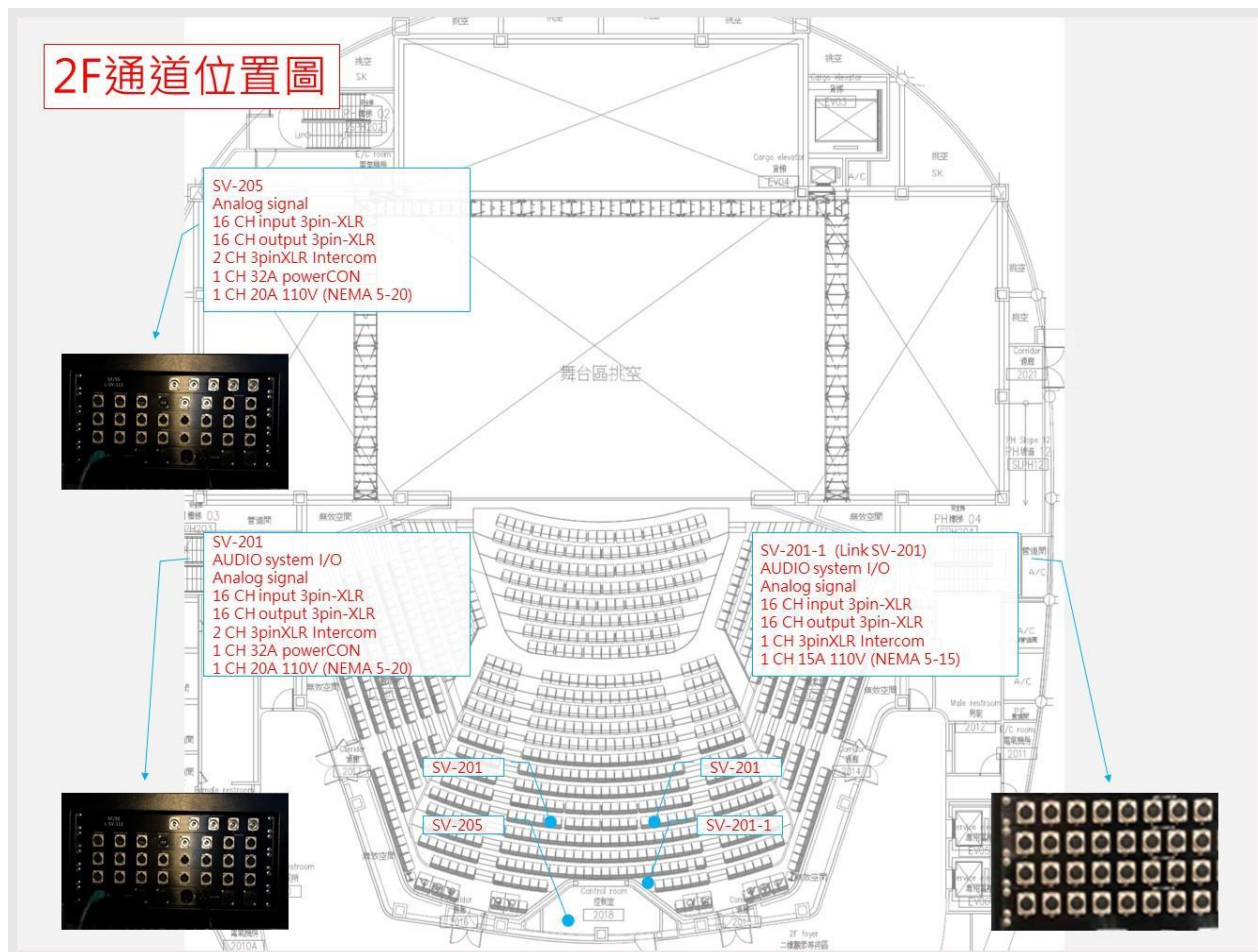
圖例 4-1.4 音響 2F 通道圖示
