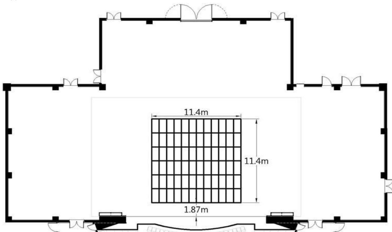
圖例 2.3-舞台陷阱位置圖
