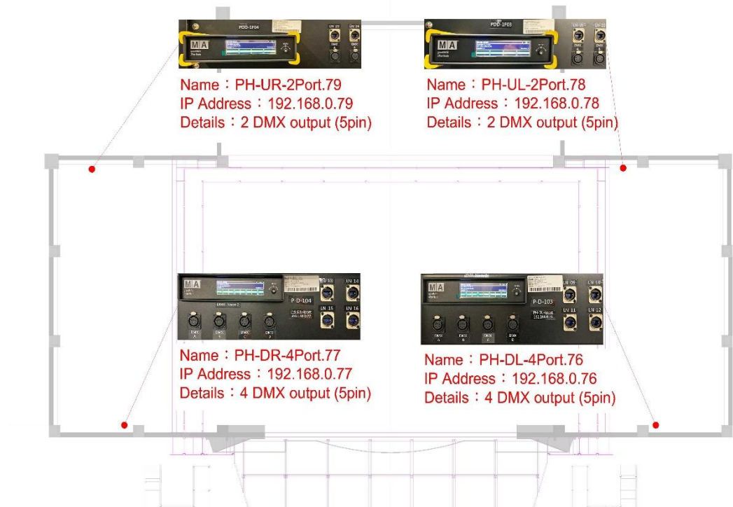
圖例 3.3.2- 舞台區 Node 位置圖
