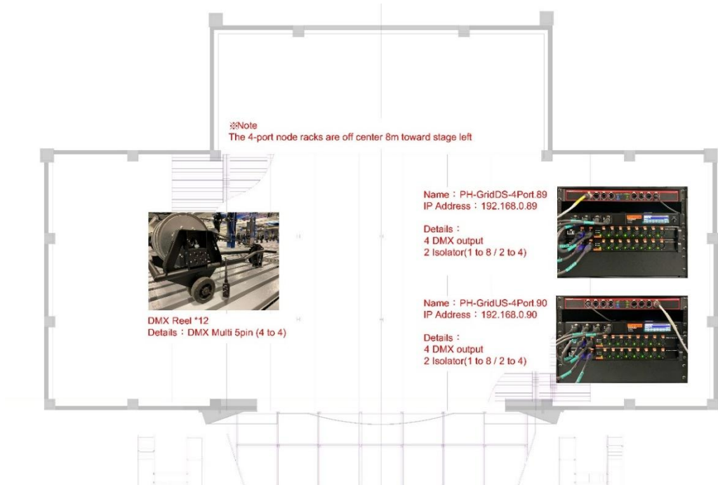
圖例 3.3.1- 頂棚區 Node 位置圖
