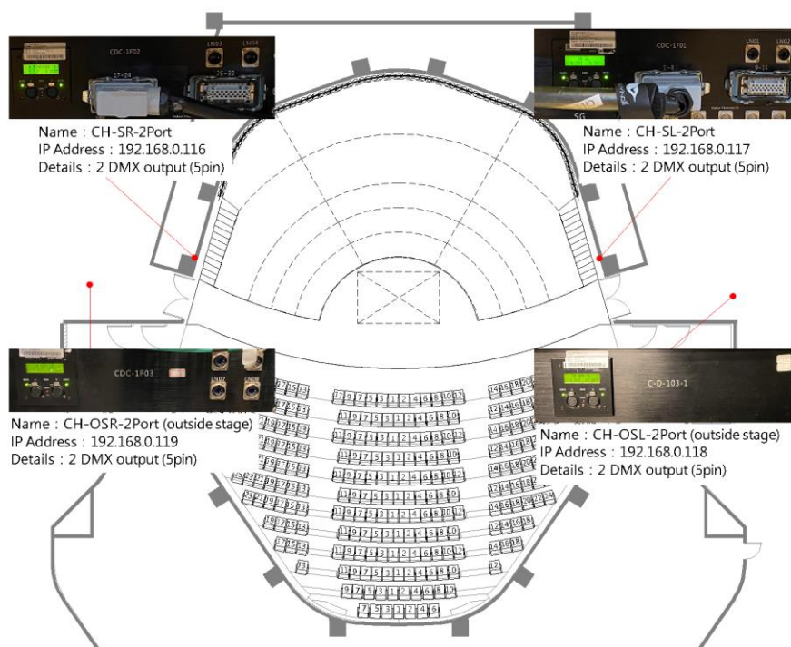
圖例 3.4.2- 舞台區 Node 位置圖
