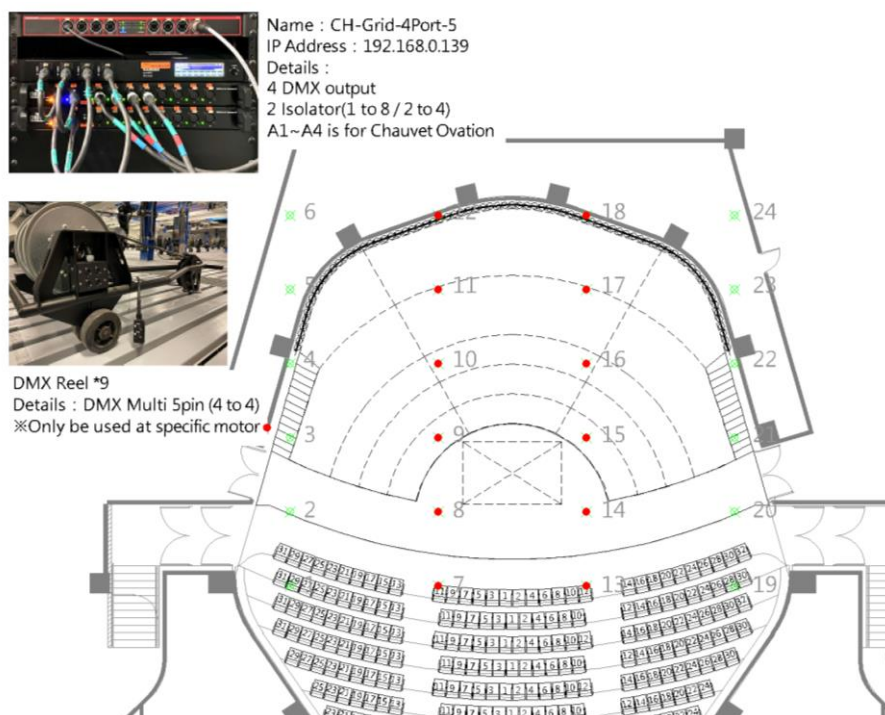
圖例 3.4.1- 頂棚區 Node 位置圖
