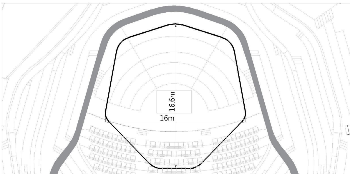
圖例 2.4-音響反射板位置圖
