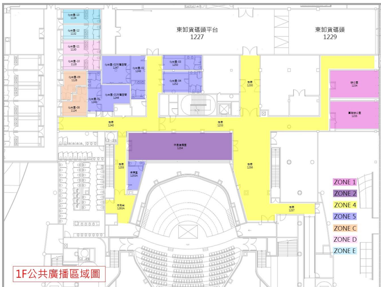
圖例 4-8.2 1F 公共廣播區域圖示
