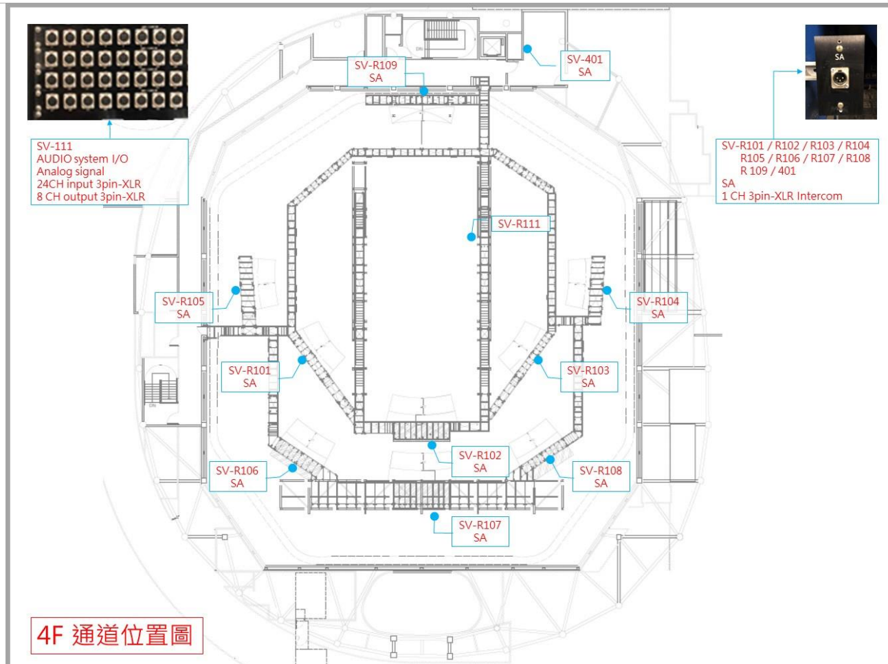
圖例 4-1.3 音響 4F 通道圖示
