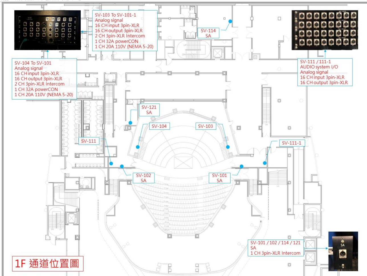
圖例 4-1.1 音響 1F 通道圖示
