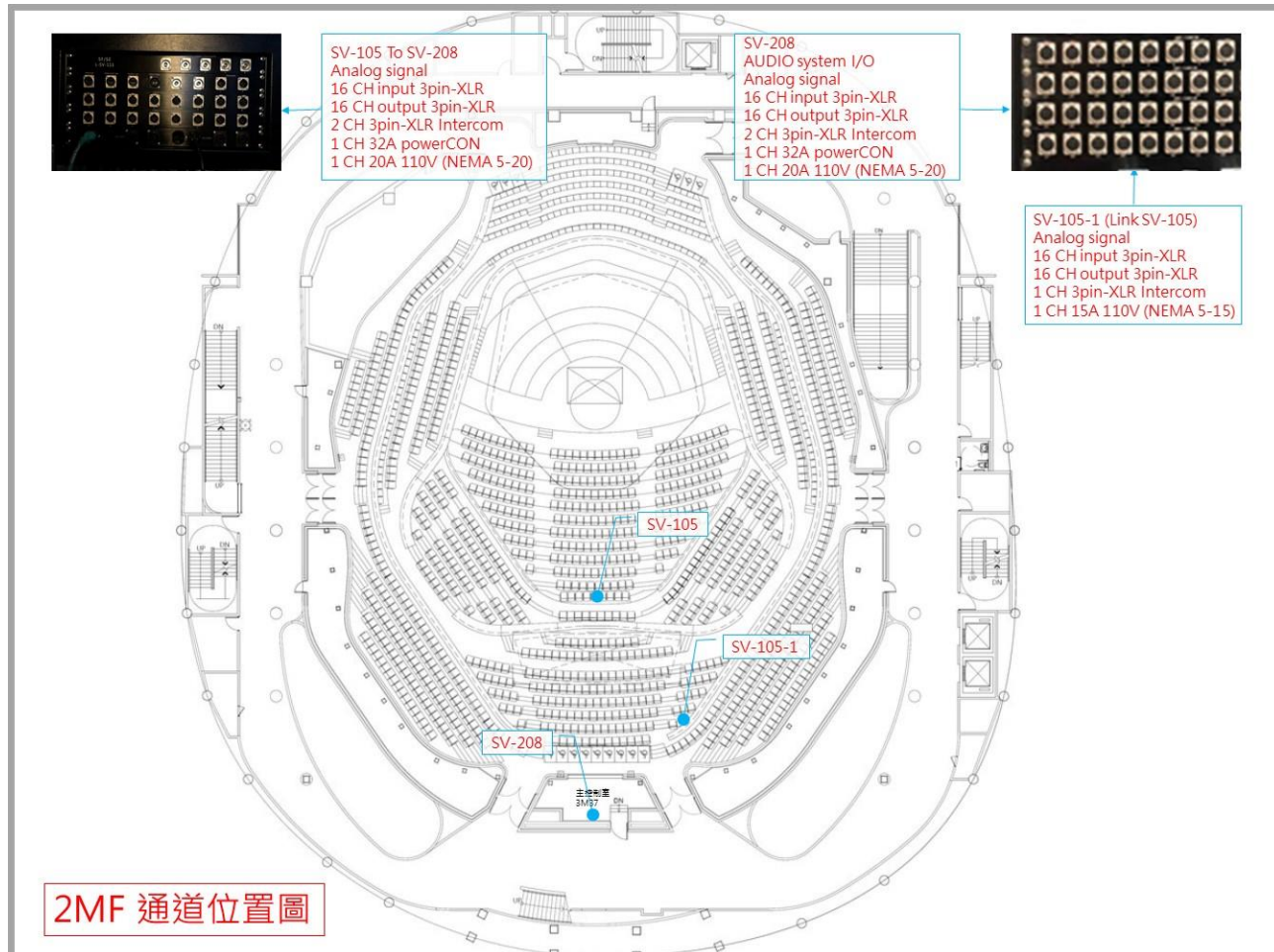
圖例 4-1.2 音響 2MF 通道圖示
