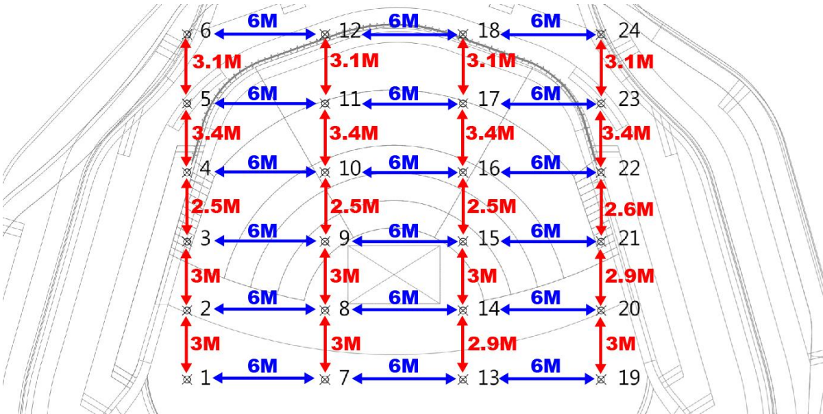
圖例 2.2 鍊條馬達位置圖
