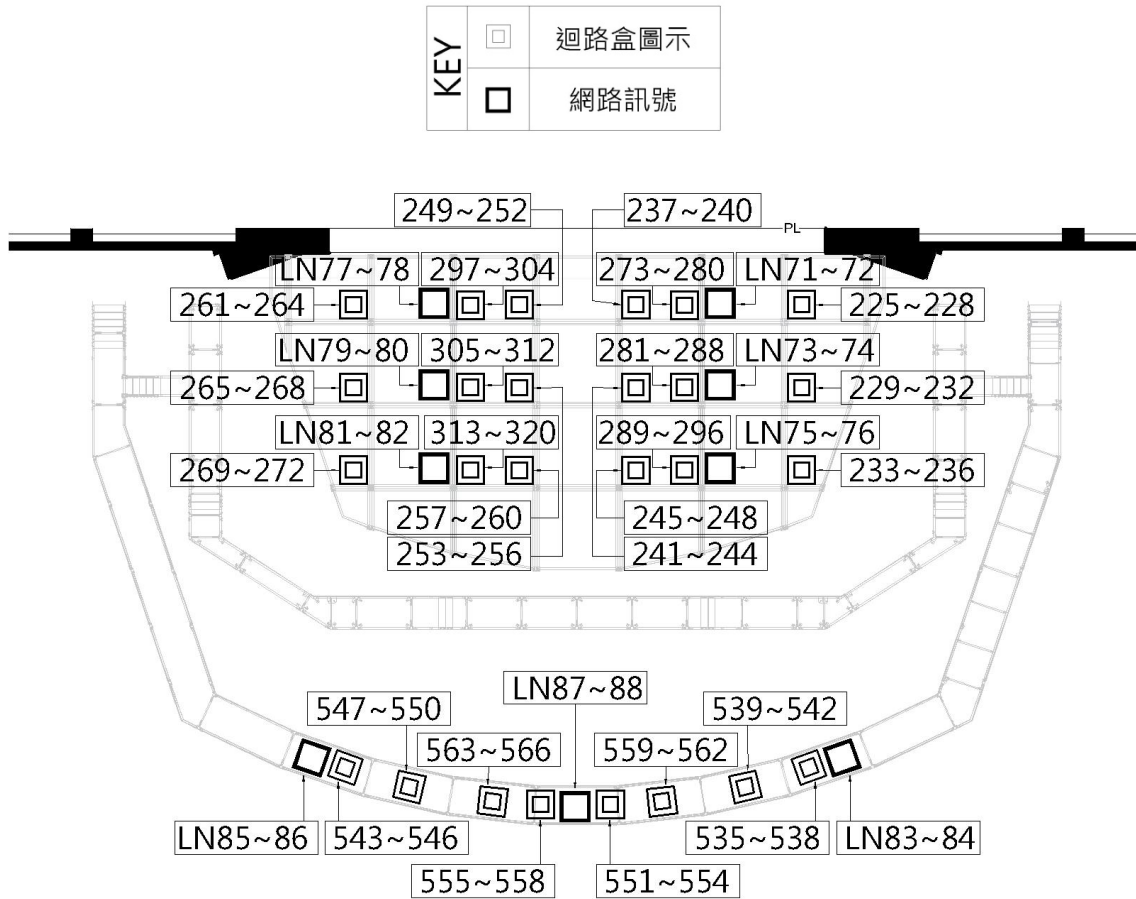
圖例 2.3.5 張力索棚架與貓道迴路配置
