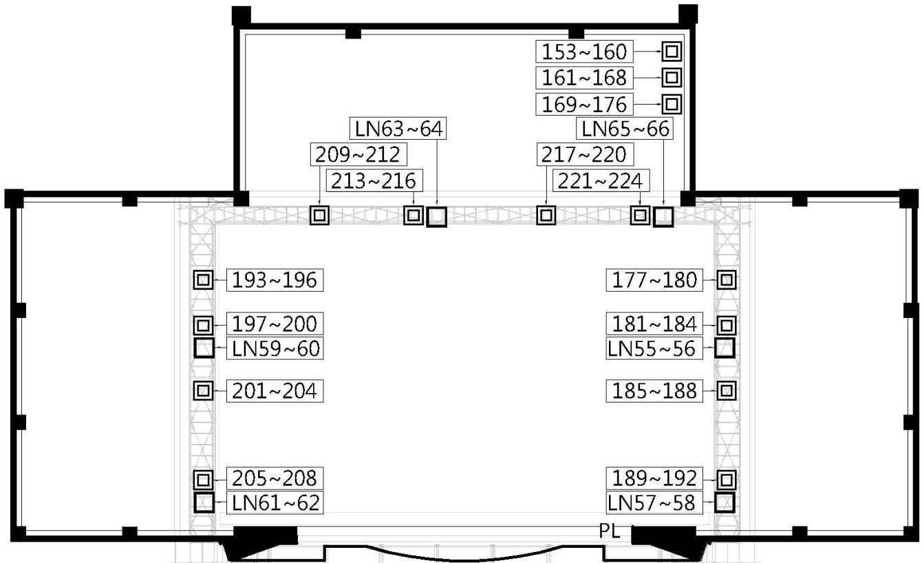
圖例 2.3.2 舞台工作廠道區迴路配置
