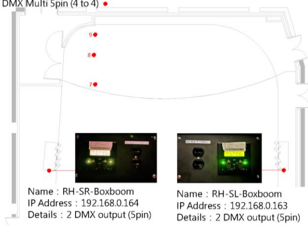
圖例 3.3.1- 頂棚及包廂區 Node 位置圖
