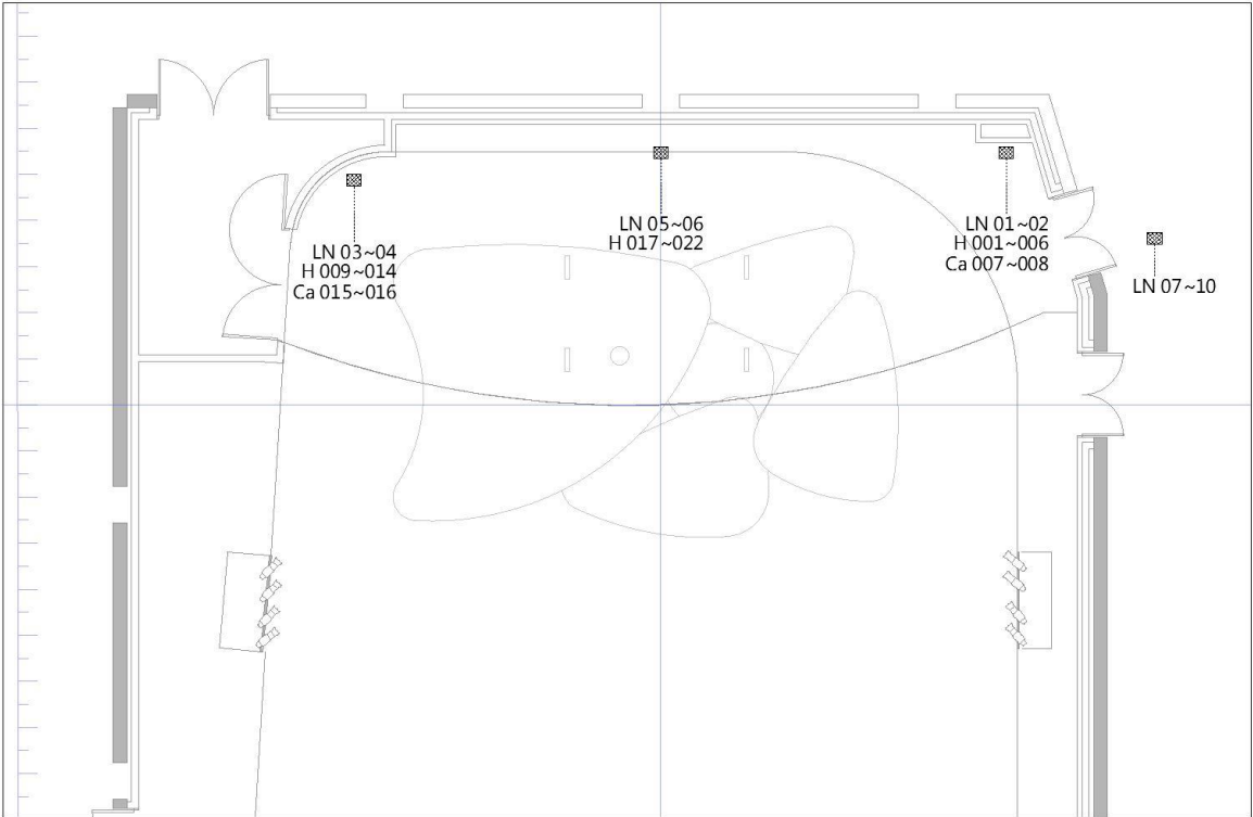
圖例 3.4.1.1- 舞台區燈光迴路配置
