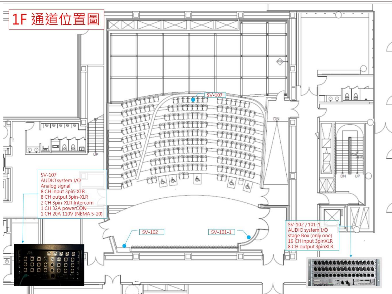
圖例 4-1.1 一樓音響通道圖示
