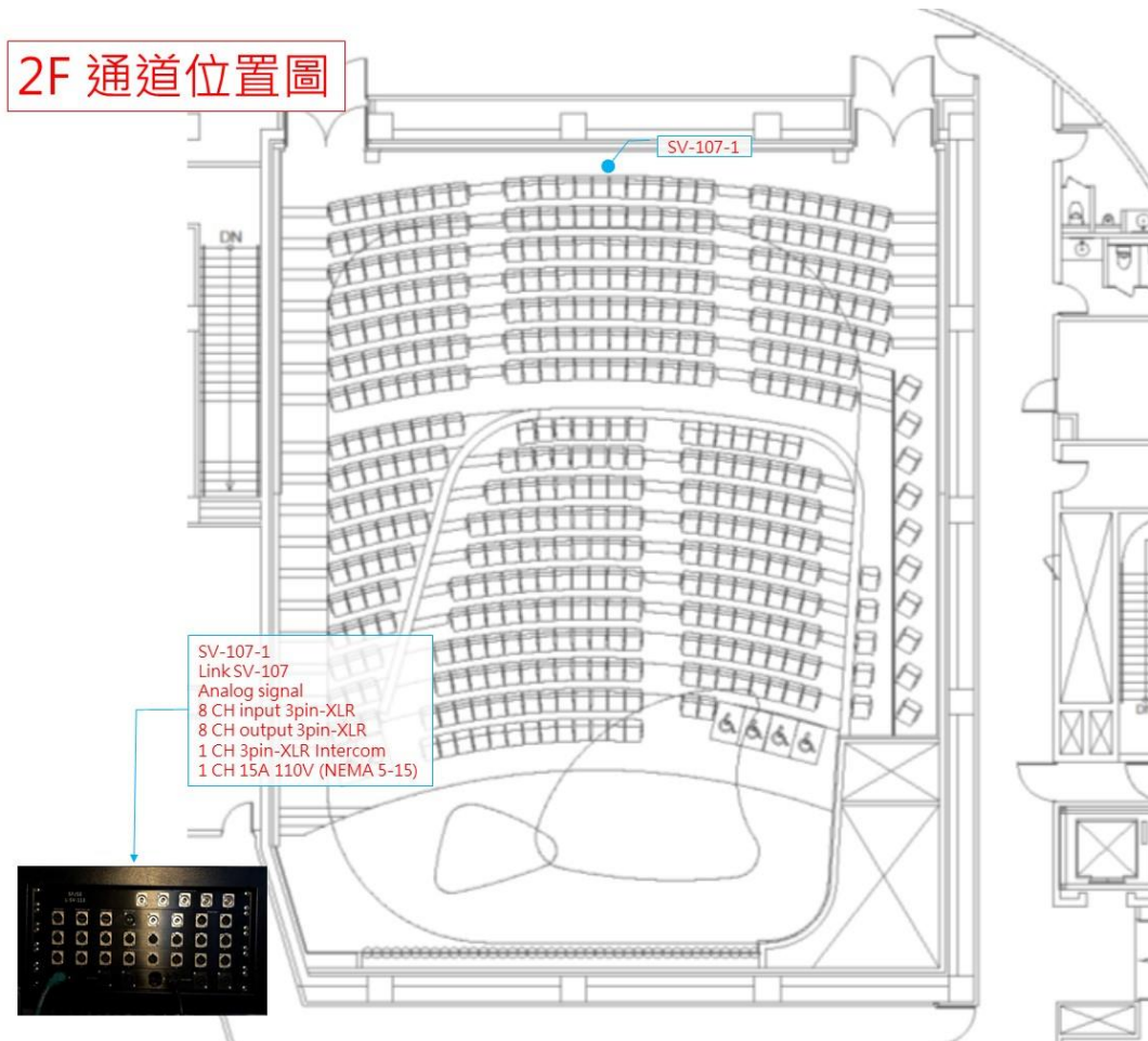
圖例 4-1.2 二樓音響通道圖示
