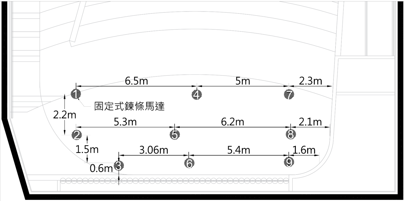
圖例 2.4 鍊條吊車位置圖
