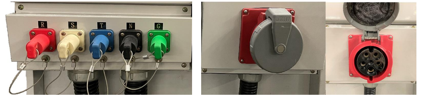
圖例 3.6- 外接電源 Camlock、CEE125 圖示
