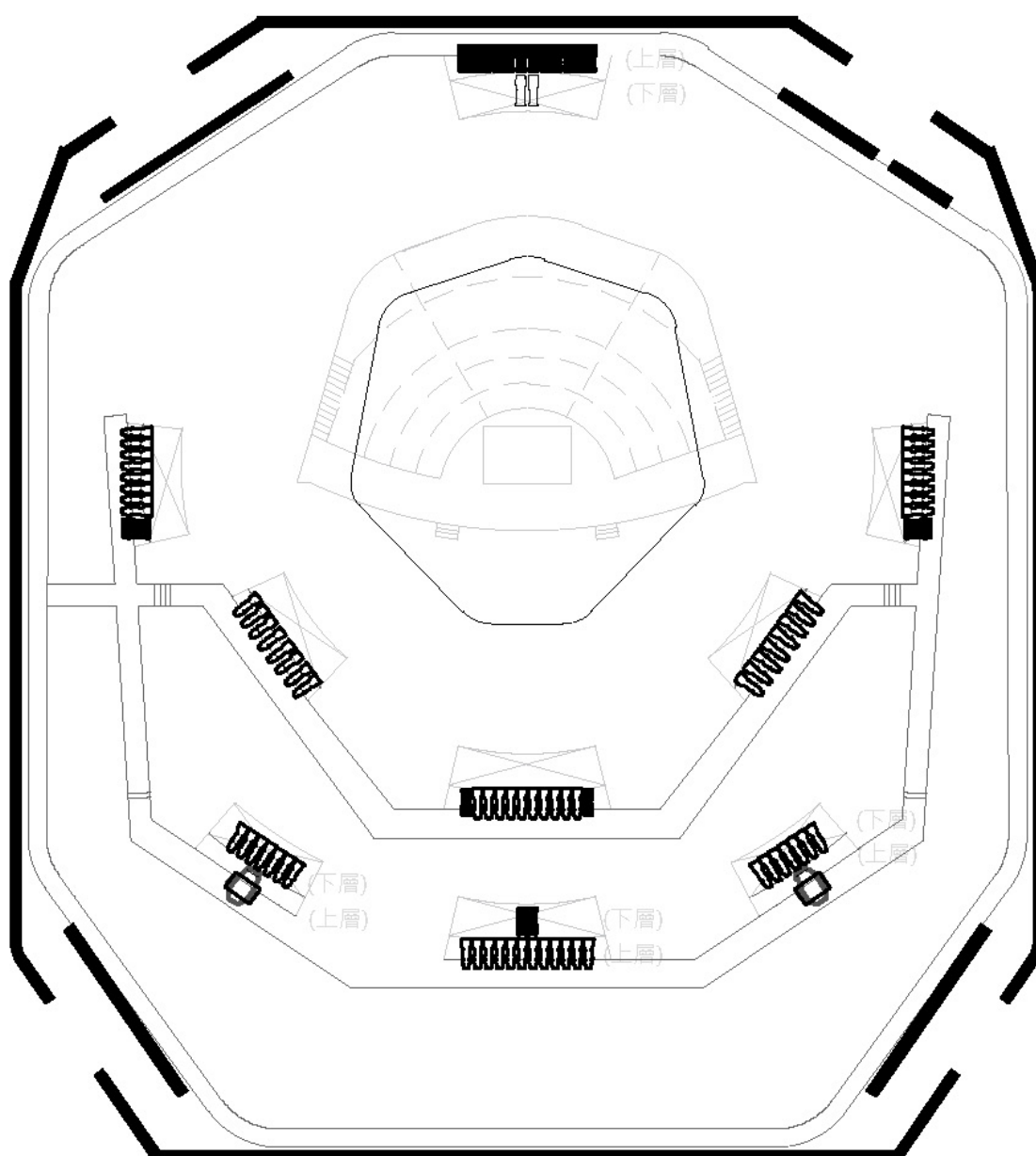
圖例 2.2 外區燈具配置圖
